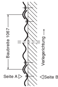
Anwendung Fassade
