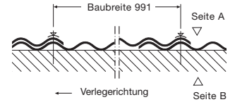
Anwendung Dach
