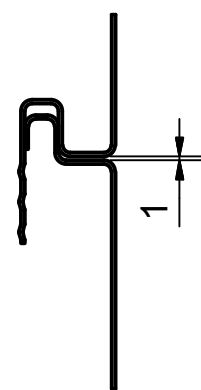
Detail Stoss/ Fugenverbindung
