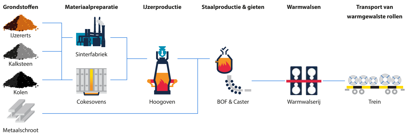
Afbeelding 1 Voorbeeld procesoverzicht
