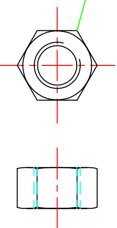
M12 Hex Nut
